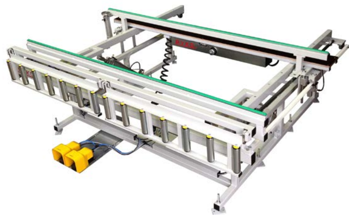
Ausführung mit Fußschaltern und Handtastern am Tisch angebracht
